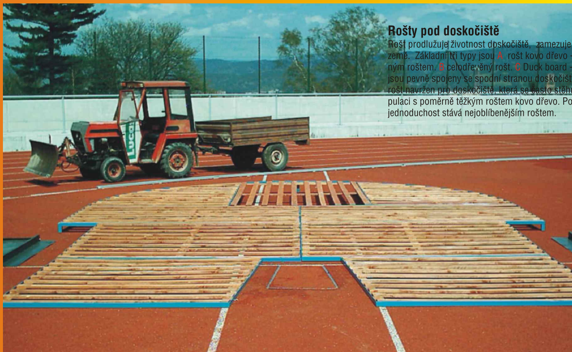
Rošt - kovo-dřevo
